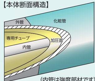
【本体断面構造】
